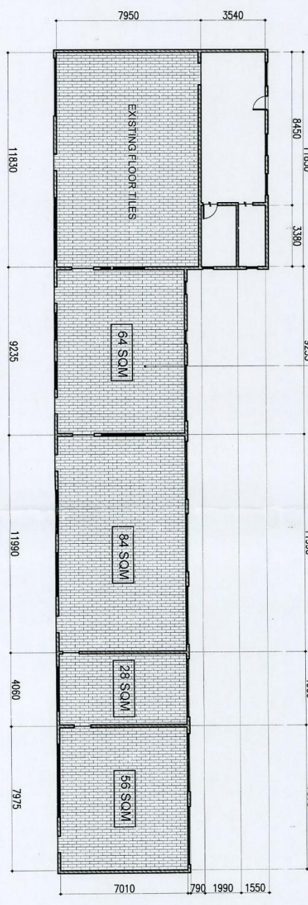
TILE LAYOUT PLAN SCALE: 1:175
