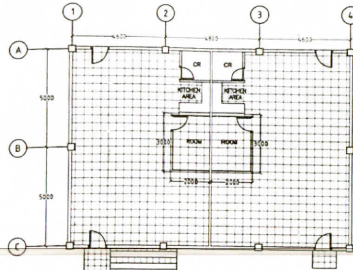
FLOOR PLAN N.T.S.
