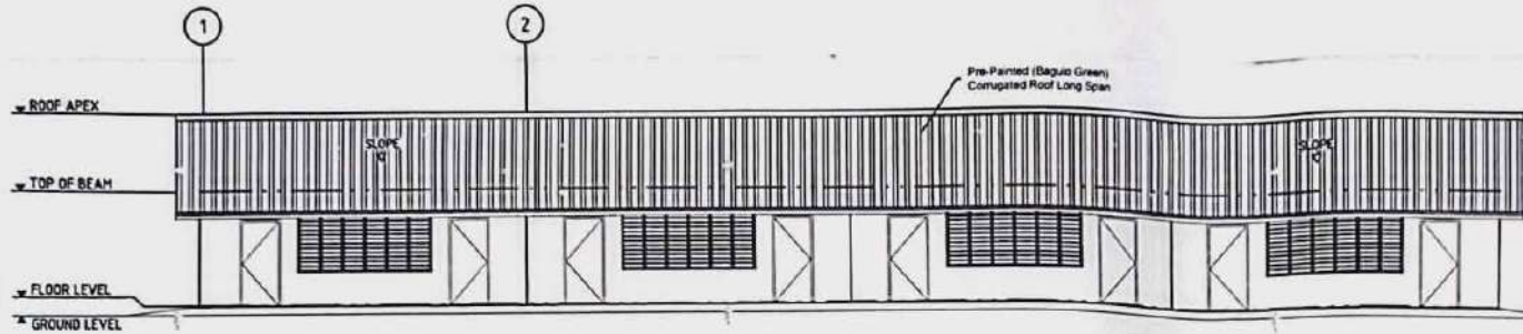
FRONT ELEVATION N.T.S.
