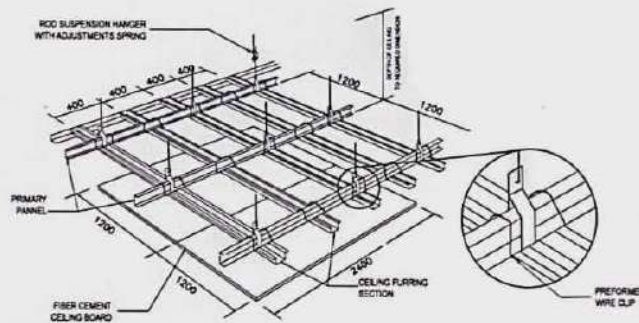
CEILING PERSPECTIVE N.T.S.
