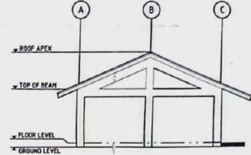
LEFT SIDE ELEVATION N.T.S.
