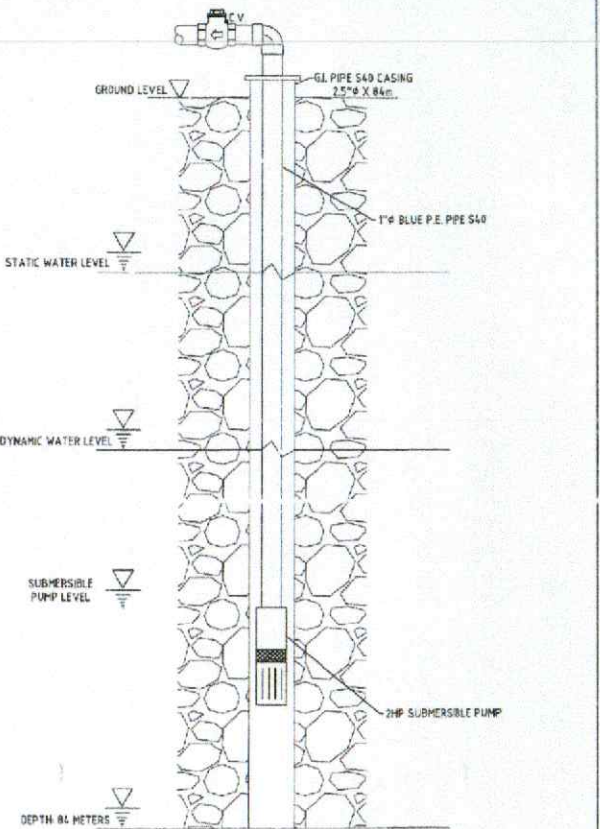
DEEP WELL DETAILS N.T.S.
