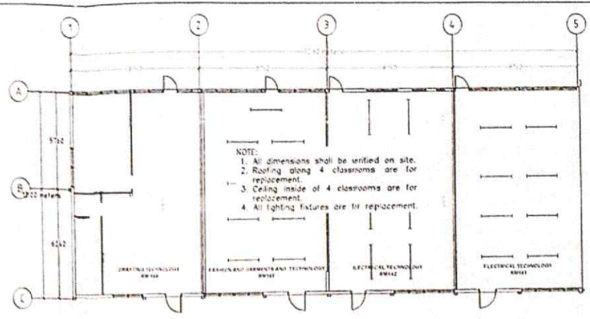
FLOOR PLAN N.T.S.
